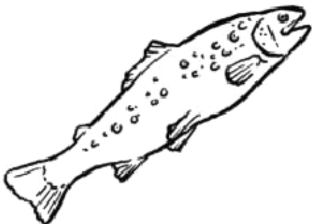
poisson
